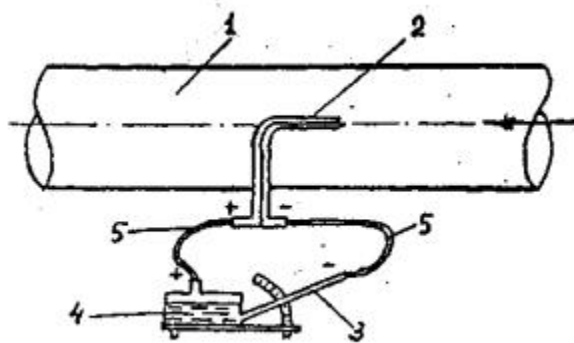
Рис.1. Схема присоединения пневмометрической трубки к микроманометру при измерении динамического давления в воздуховоде:
