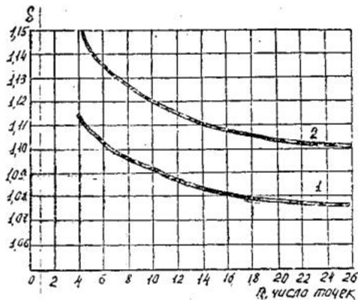
Рис. 2. График поправочных коэффициентов на величину расхода, воздуха по воздуховоду при измерении по методу равноотстоящих точек:
