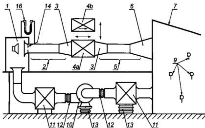
б) Испытательная установка с использованием реверберационного помещения
