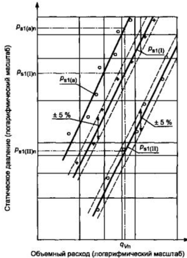
Рисунок 9 - Требования к отношению расход/давление (график статического давления и соответствующего расхода в плоскости I)
