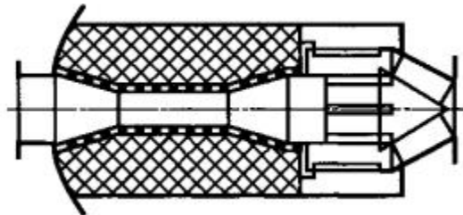
Рисунок 1 - Примеры глушителей, лист 1
