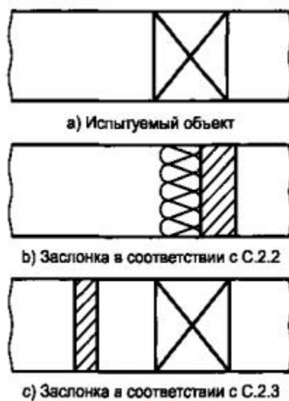
Рисунок С.2 - Устройство испытательного стенда для определения предельных вносимых потерь
