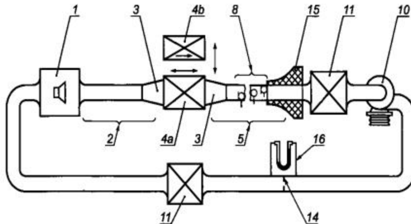
а) Испытательная установка для измерений в воздуховоде
