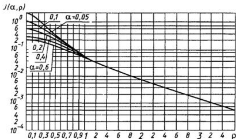
Рисунок Б.2 - График для определения функции J(a, r) , описывающей поле отраженного звука в несоразмерном помещении
