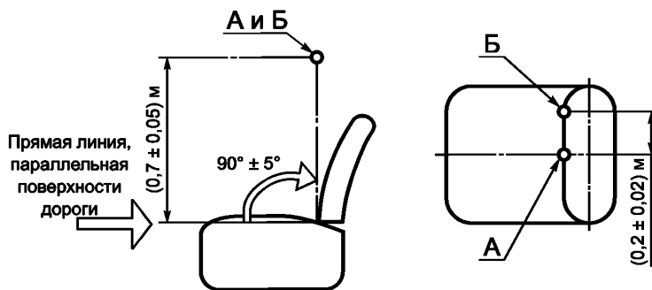
Рисунок 1 — Положение микрофона относительно сиденья
