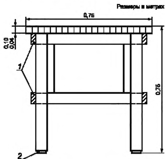
Рисунок Е.1 — Пример конструкции испытательного стола
