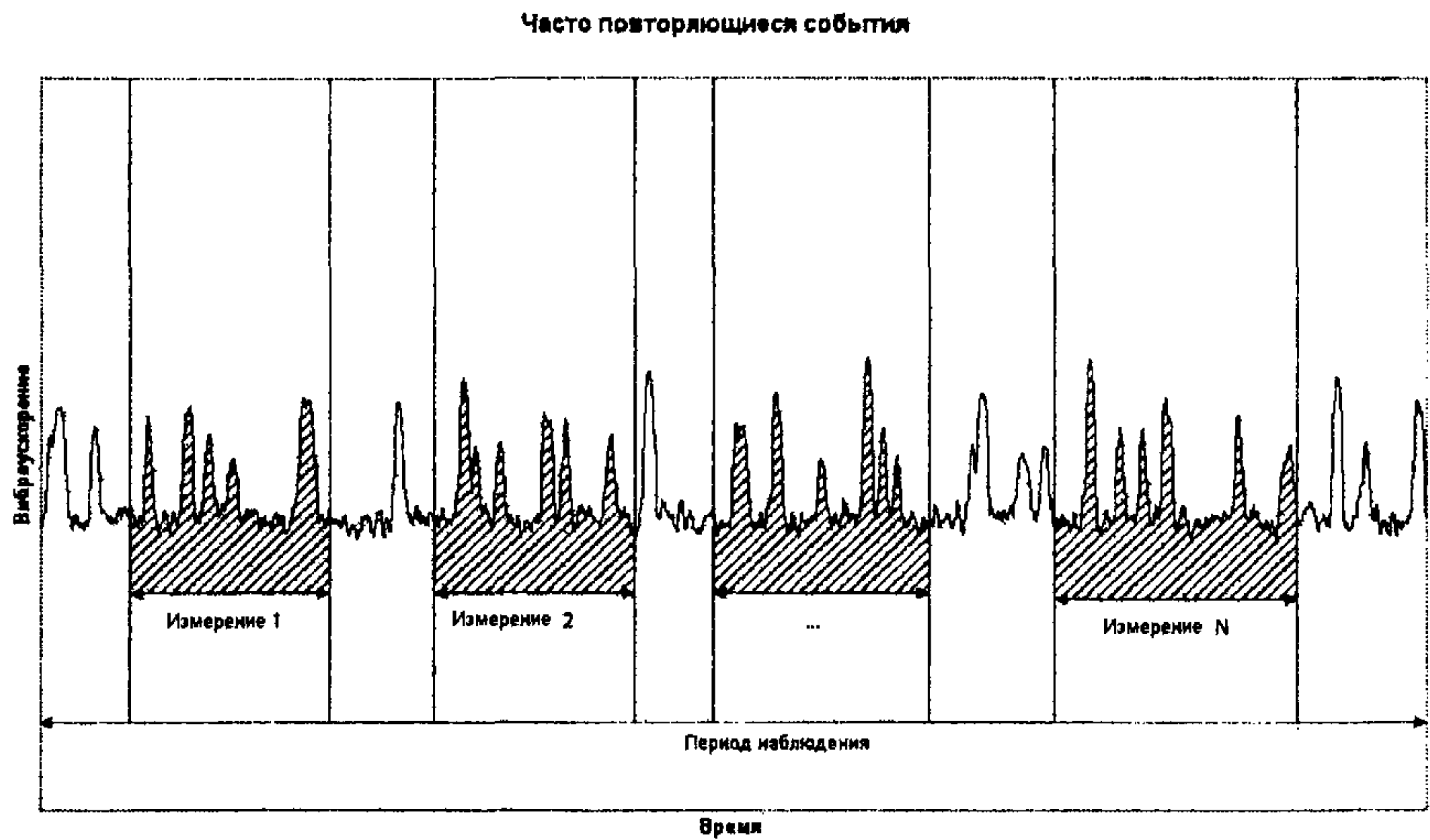
Рис. 3. Периоды контроля, наблюдения и измерений в случае часто повторяющихся вибрационных событий
