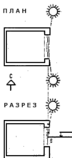
Рис.1. Схема определения расчетной точки для окна
