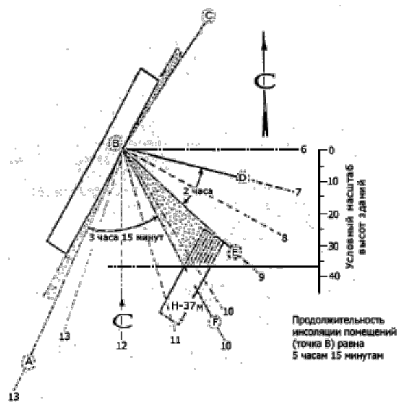
Рис.5. Схема определения инсоляции
